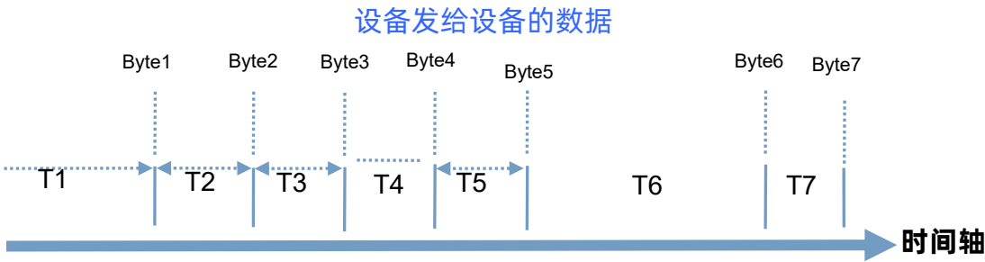
图 5 切换指令模式时序
