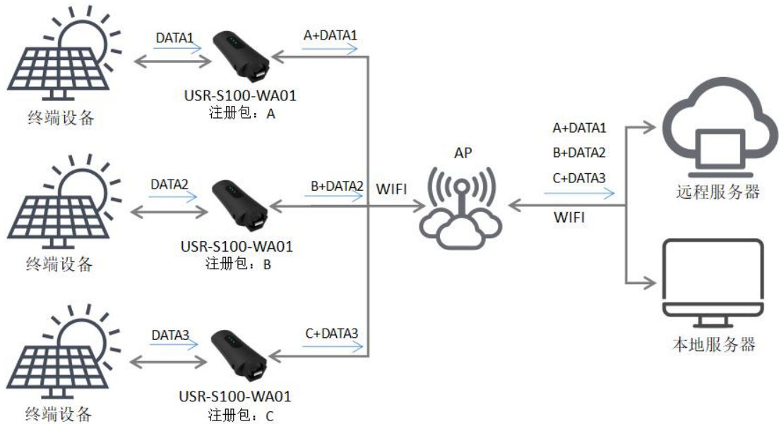
图 8 注册包功能框图
