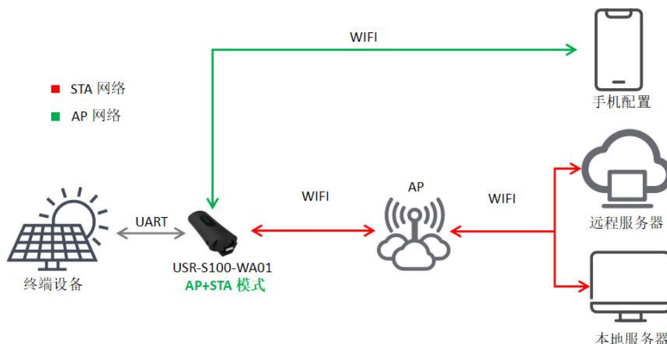
图 3 AP+STA 模式组网
