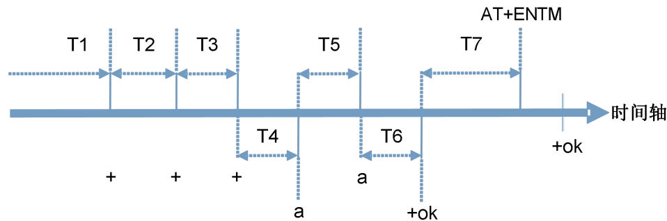
图 13 切换指令模式时序
